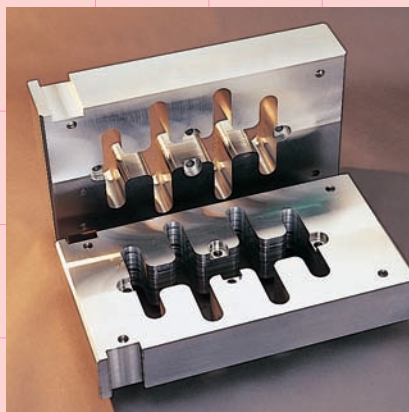
ベースプレート溝加工
